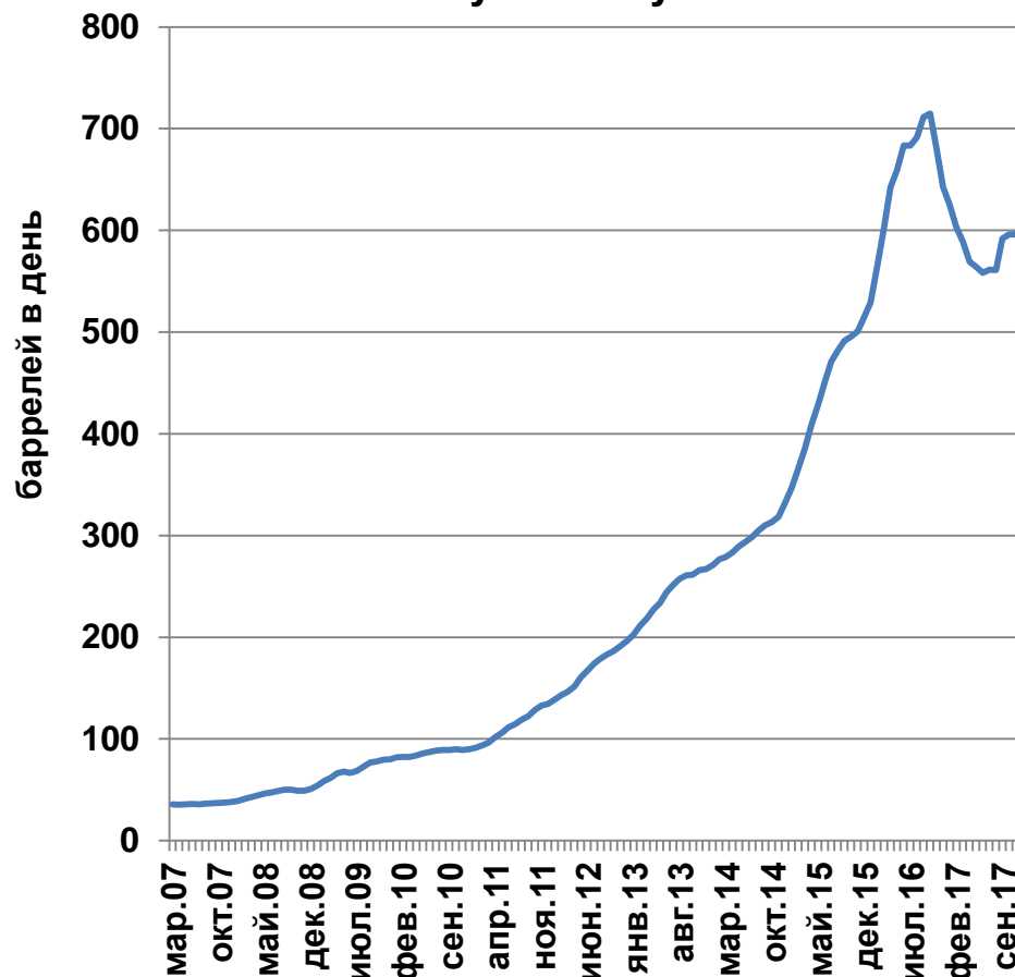
Добыча нефти и конденсатов на основных сланцевых формациях США из новых скважин в расчете на одну буровую установку
