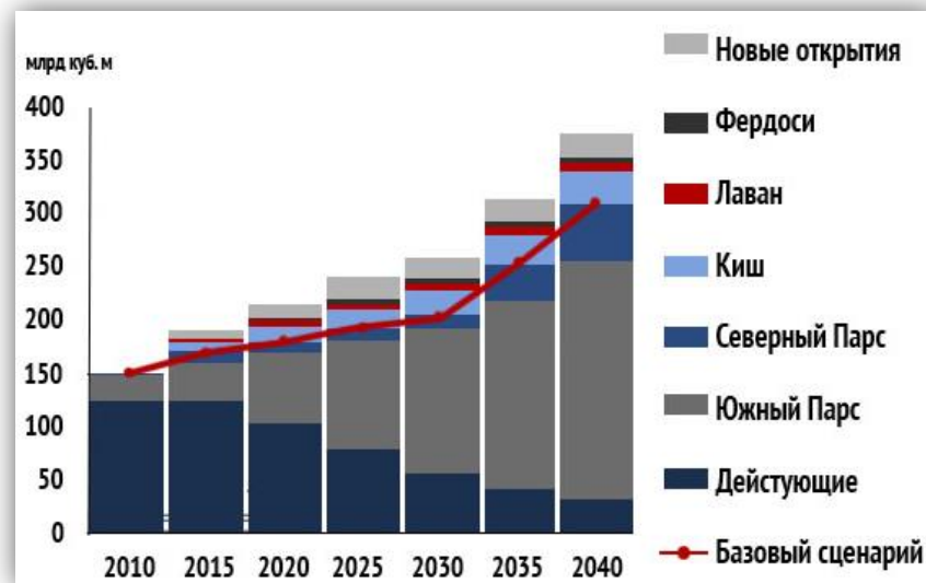
Рисунок 2. Прогноз добычи газа в Иране
